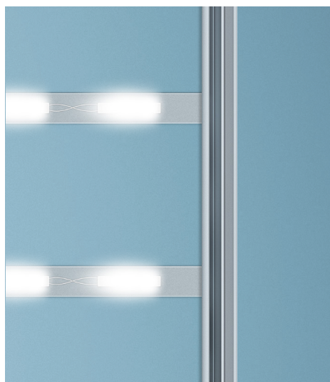
Lightframe mit LED-Hinterleuchtung Tiefe: ca. 150 mm Material: Aluminium silber eloxiert Tuchführung: einseitig bespannbar Anwendung: Wandmontage
